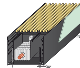
Bodenkanalheizung
