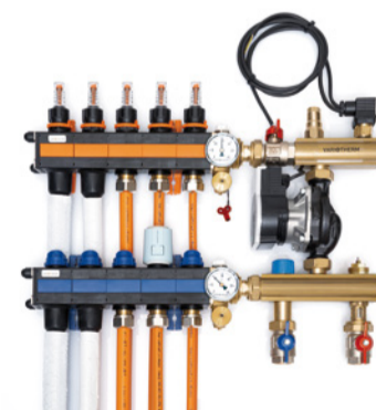
Vario-PumpenVerteilerstation 5.0
